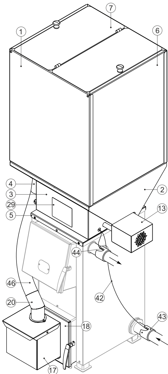
Рис. 1. Конструкция АПГ-25
