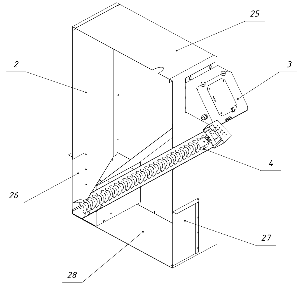
Рис. 36 Бункер с податчиком пеллет и блоком управления.
