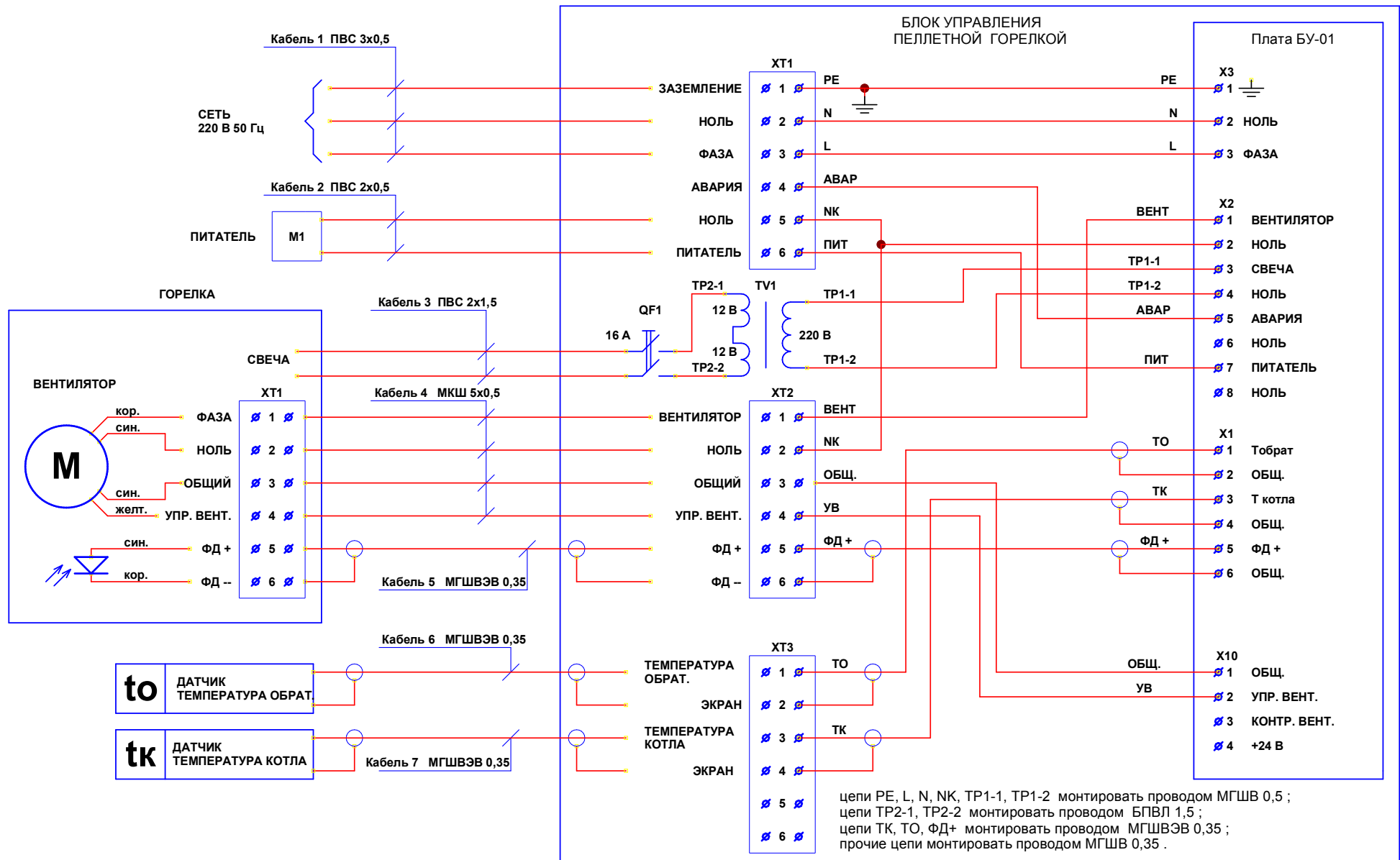
Рис. 8. Схема монтажная.
