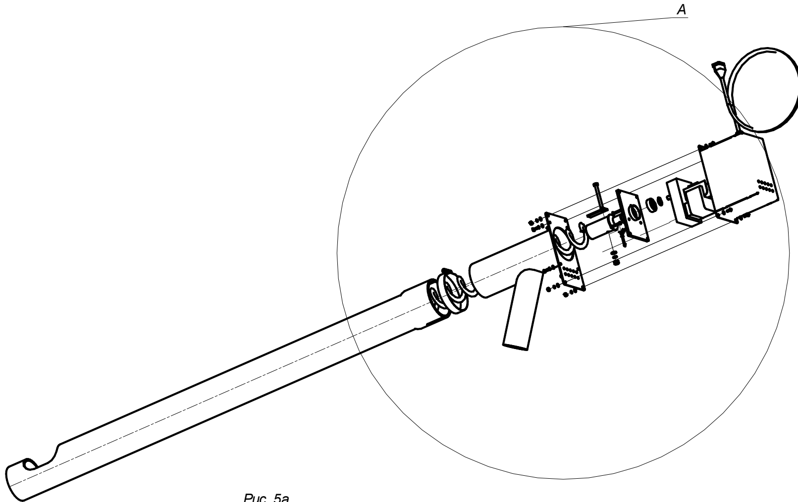
Рис. 5а Податник пеллет.
