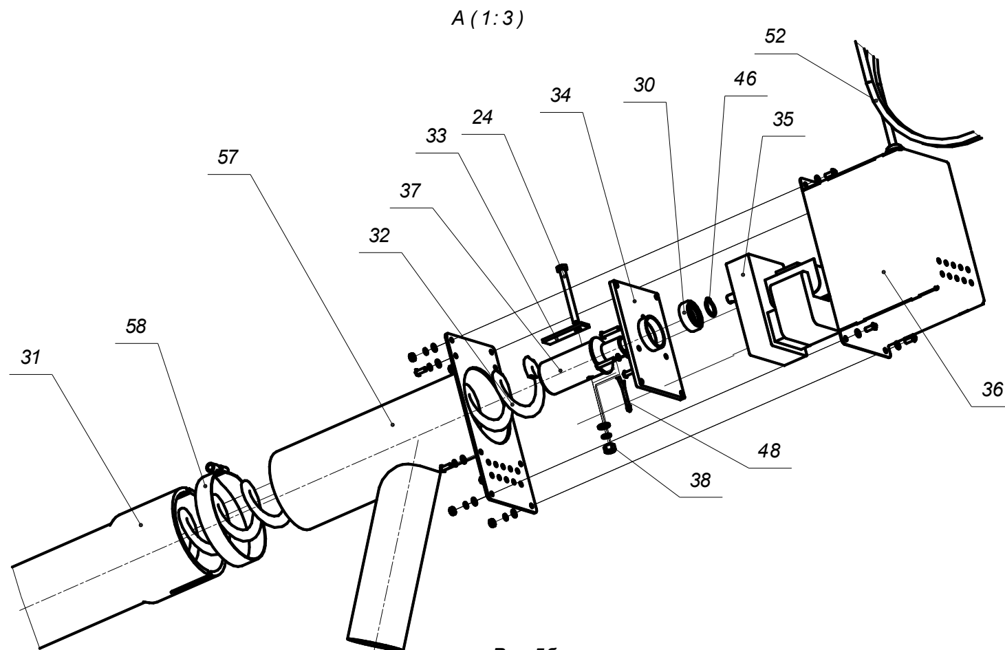
Рис. 56 Податчик пеллет
